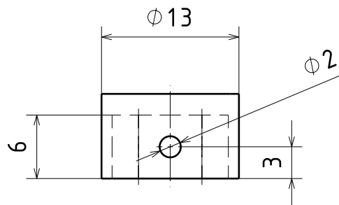
Kolben M 2:1
