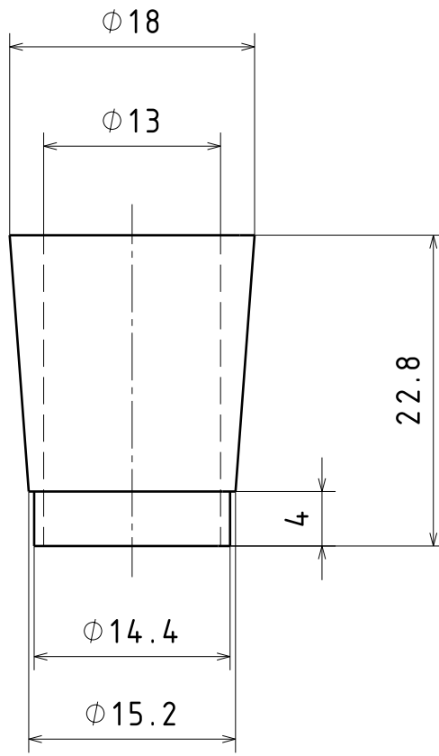
Zylinder M 2:1
