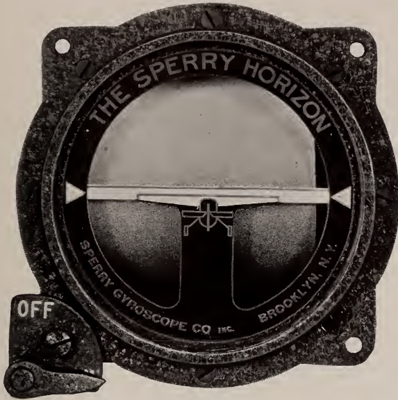
Fig. 6—Sperry Horizon.
